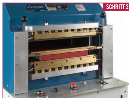
Wenn die korrekte Position gefunden ist, wird der hydraulische Presszyklus ausgelöst.
