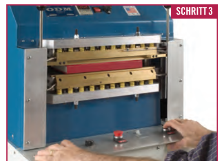
Das Buch wird ordentlich zwischen zwei Stahlplatten gepresst und der Falz wird durch die beheizten Formeisen "eingebrannt".
